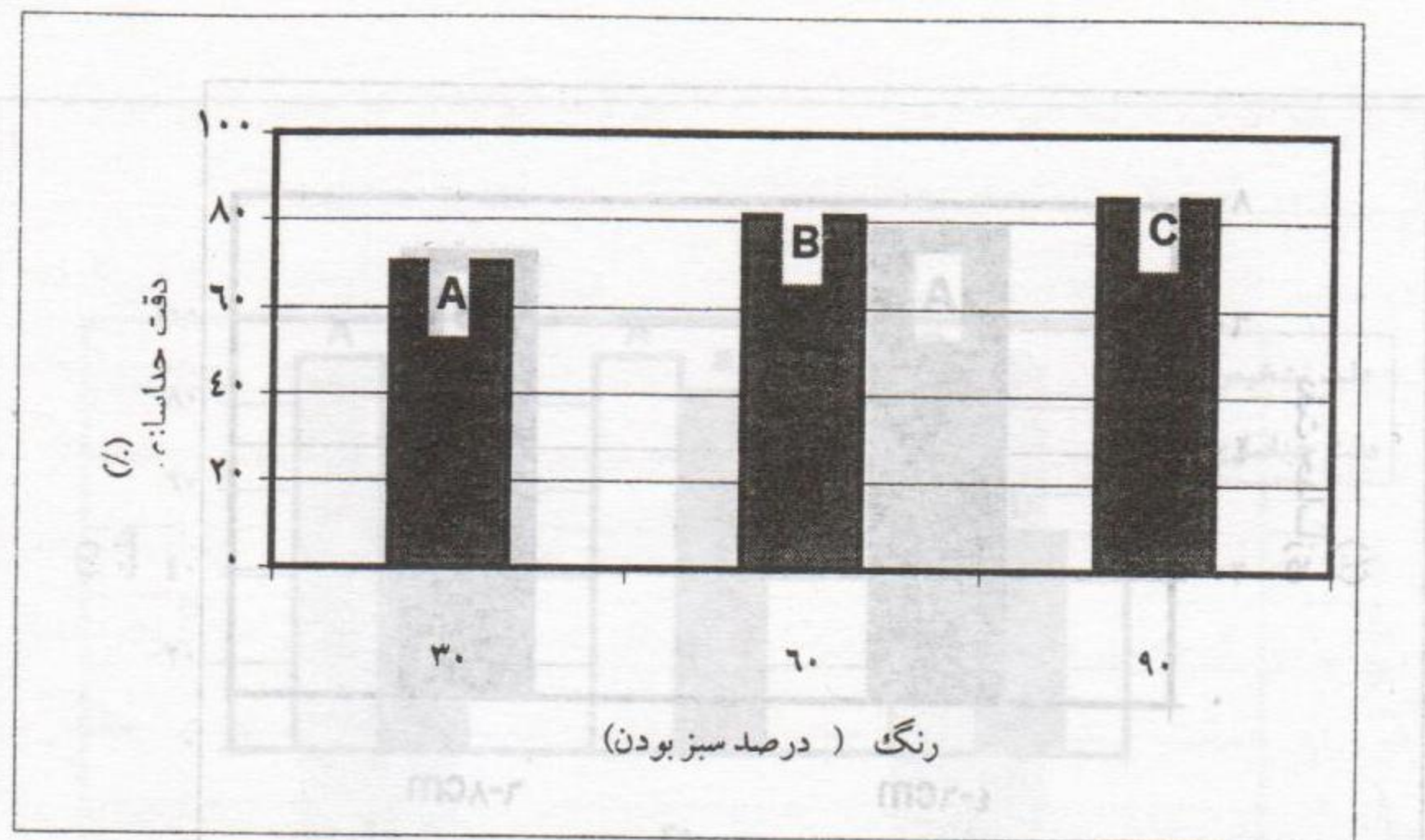
شکل ۲- نمودار تاثیر درصد سبز بودن گوجه‌های غیر قرمز بر دقت جداسازی دستگاه
