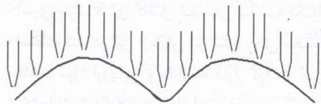
شکل ۲- شیار بازکنهایی که حالت جوی و پشته ای دارند
