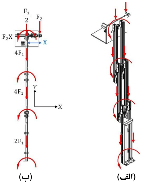
شکل (۲) نیروها و گشتاورهای وارد بر بازوهای ربات. الف) نمایش سه بعدی، ب) نمایش دو بعدی. Figure (3) Forces and torques on the robot manipulator. A) 3D display, b) 2D display.
