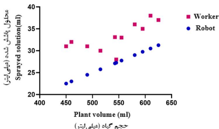
شکل (۱۱) مقایسه مقدار محلول پاشش شده توسط ربات و کارگر به ازای حجم بوته
