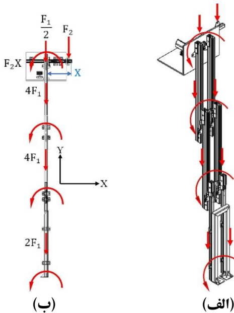
شکل (۲) نیروها و گشتاورهای وارد بر بازوهای ربات.
