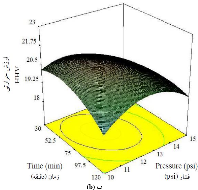
شکل (۲) نمودار دو بعدی (الف) و سه بعدی (ب) اثر پارامترهای زمان ماند، فشار و نسبت باگاس به میزان HHV Figure (2) 2D (a) and 3D (b) representations of the effect of residence time, pressure and the ratio of BAGASSE on the HHV
