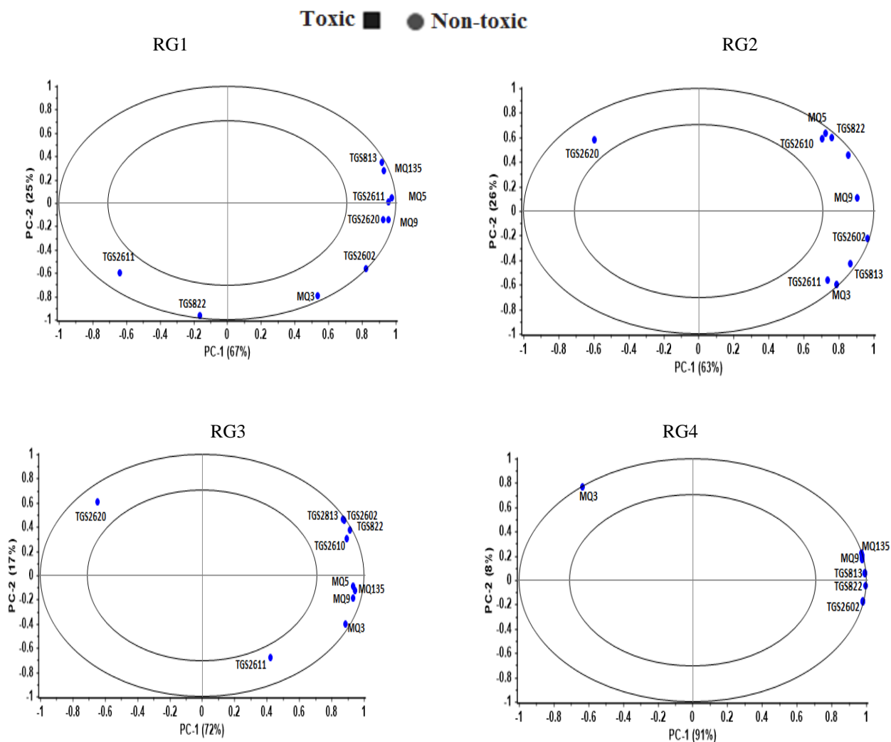
شکل (۶) نمودار لودینگ PCA در تشخیص آبلووی ارگانیک و غیرسمی ( PC-1:مولفه اصلی اول و PC-2:مولفه اصلی دوم) Figure (6) PCA Loading diagram for detection of Organic and Inorganic sour Cherries (PC-1:First analysis component and PC-2:Second analysis component)
