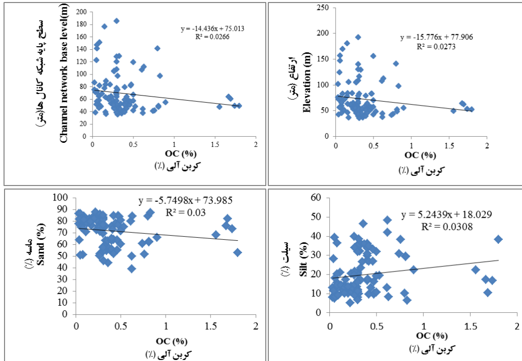
شکل (۳) ضریب همبستگی بین برخی متغیرهای کمکی و کربن آلی خاک
