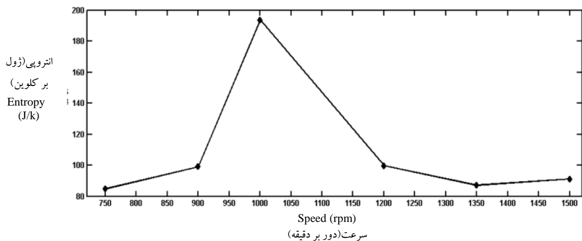
شکل (۵) مقادیر انرژی استخراج شده از سیگنال ها (سرعت دور بر دقیقه)
