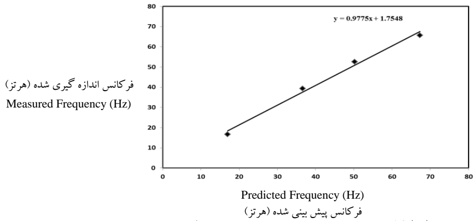
شکل (۱۳) فرکانس های طبیعی پیش بینی شده و اندازه گیری شده
