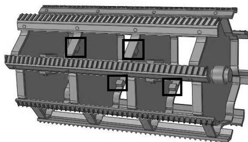
شکل (۱۲) موقعیت نصب جرم‌ها جهت اصلاح سازه
