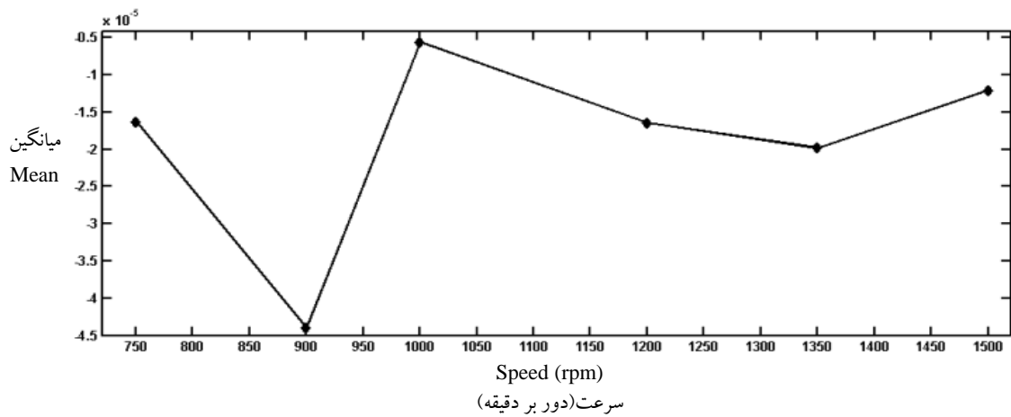
شکل (۸) مقادیر میانگین استخراج شده از سیگنال‌ها Figure (8) Mean values extracted from the signals
