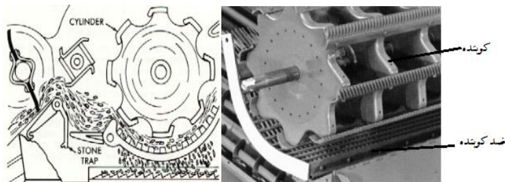
شکل (۱) واحد کوبش کمباین برداشت غلات
