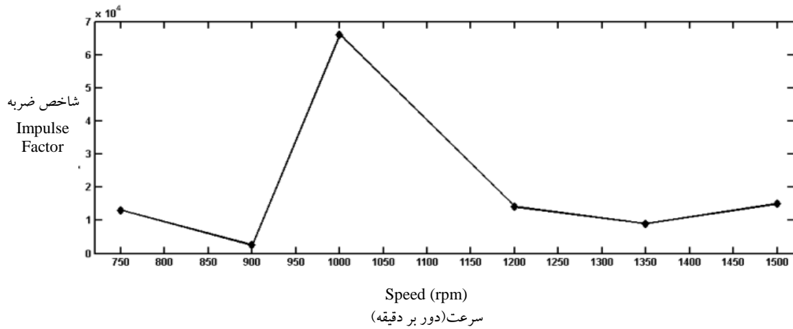
شکل (۷) مقادیر فاکتور ضربه استخراج شده از سیگنال‌ها Figure (7) Impulse factor values extracted from the signals
