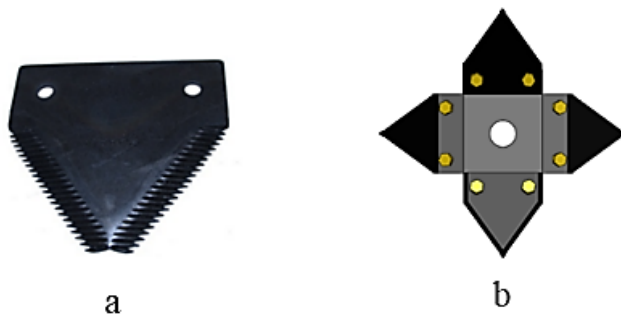
شکل (۵) (a) تیغه مورد استفاده، (b) نحوه نصب تیغه‌ها بر روی یک فلنج
